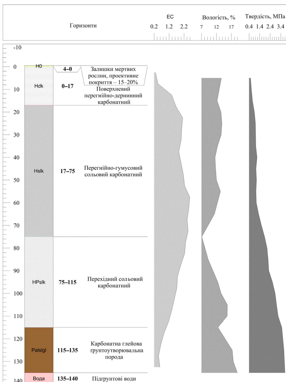
Рис. 6. Профіль алювіального лучно-болотного суглинкового карбонатного ґрунту
