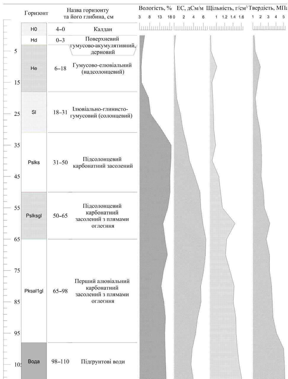
Рис. 4. Профіль алювіального лучного високосолончакуватого сильнозасоленого глибококарбонатного середнього стовпчастого ґрунту
