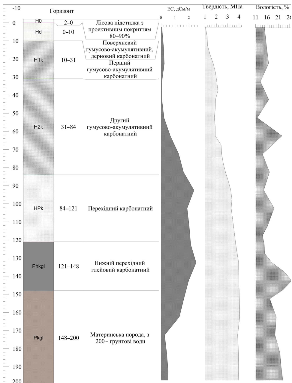
Рис. 7. Профіль дерново-лісового чорноземоподібного глибокого глейового карбонатного поверхнево-засоленого ґрунту
