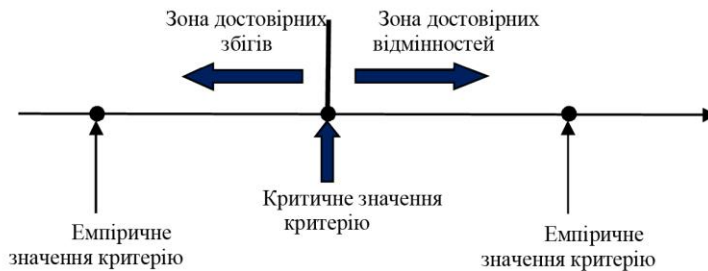
Рис. 1. Схема застосування статистичного критерію
