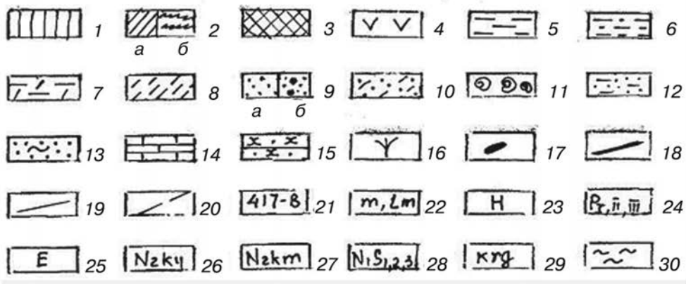
Рис. 1. Геологічний розріз Бердянської коси
