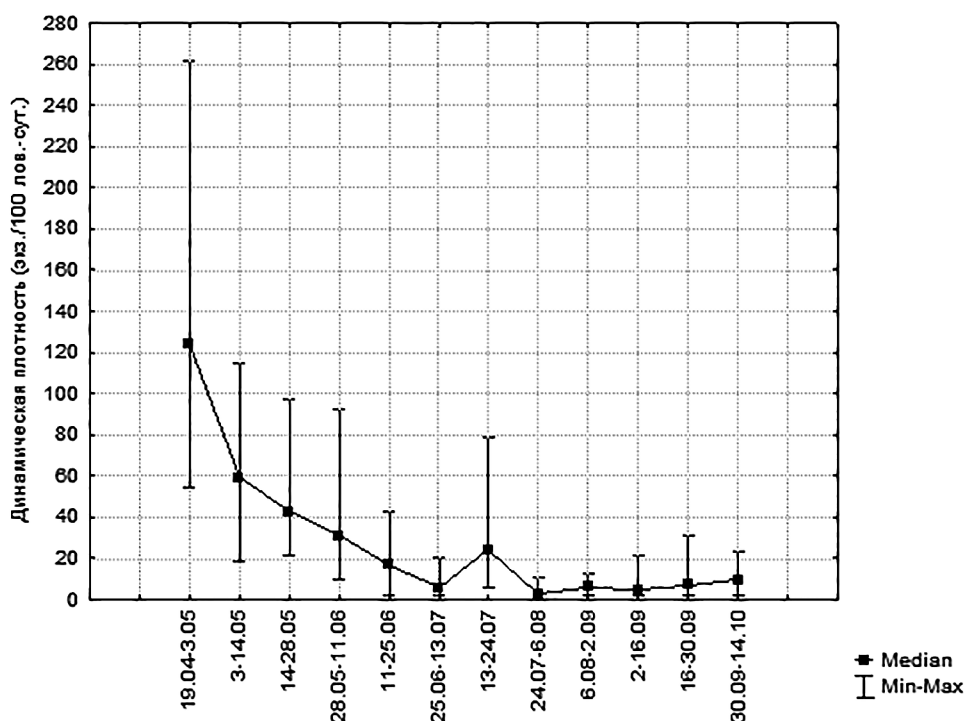
Рис. 1. Сезонное изменение динамической плотности пауков участка рекультивации (показана медиана, максимальное и минимальное значения)
